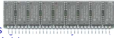
SIPP-Modul mit seinen 30 pin-förmigen Anschlüssen und einer Datenbreite von 8 Bit (IMM): PS/2-Module
